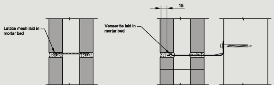
LATTICE MESH
